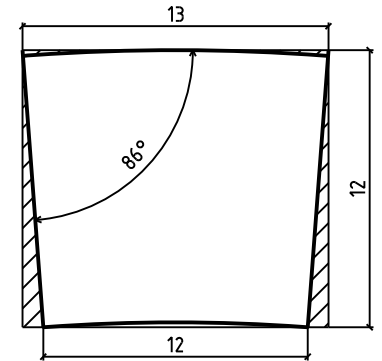
Detalle 1 Esc. 3 : 1
